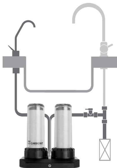
Einbauschema DUO Comfort
