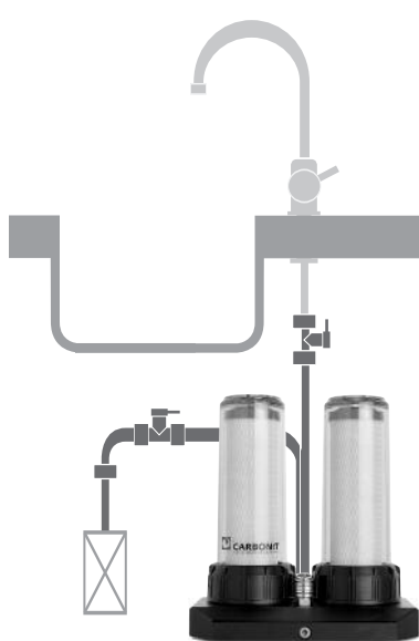
Einbauschema DUO Classic / DUO Clario
